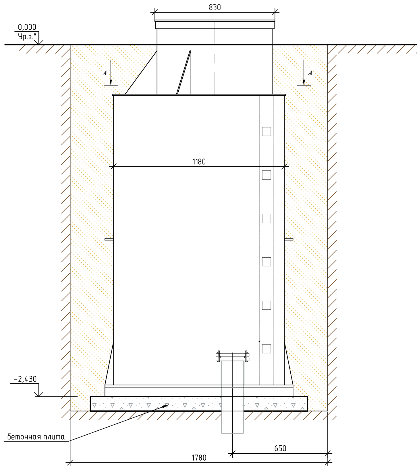
Вид спереди
